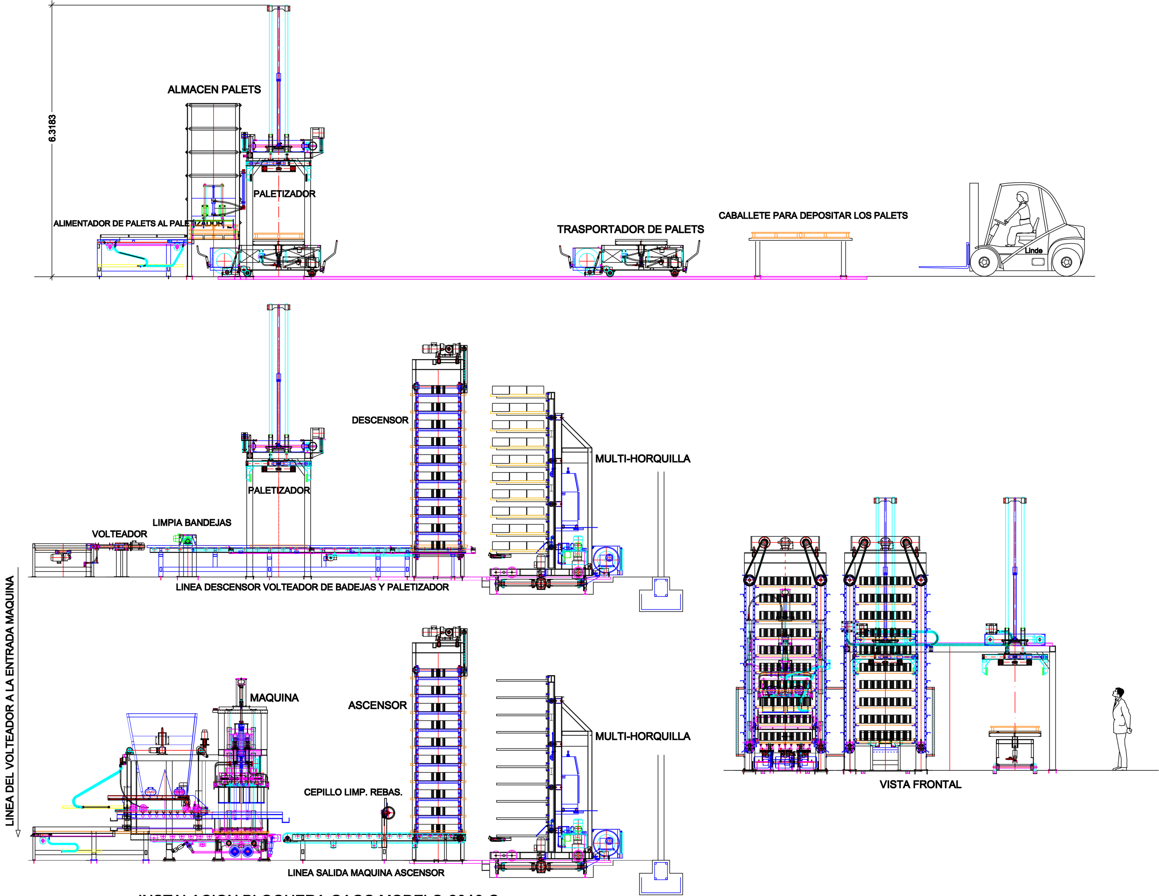
INSTALACION BLOQUERA GAGO MODELO 2013 C
